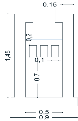
Figure 10: Coupe frontale à la sortie du premier compartiment à flux ascendant
