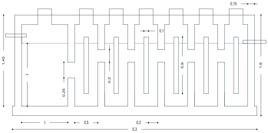
Figure 8: Vue de profil du RAC classique dimensionné
