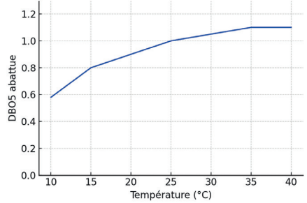
Figure 4 : Effet de la température sur le taux d'abattement de la DBO5 dans le RAC
