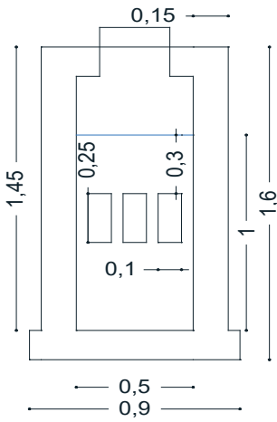
Figure 9: Coupe frontale à la sortie du compartiment de décantation
