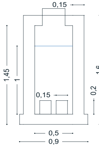
Figure 11: Coupe frontale à la sortie des chicanes
