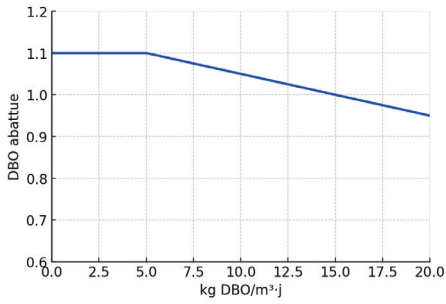
Figure 1 : Abatement de la DBO5 en cas d'une surcharge organique du RAC
