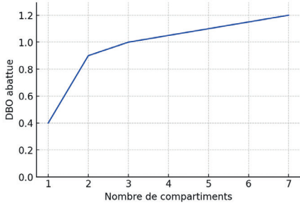
Figure 3 : Effet du nombre des compartiments sur le taux d'abattement de la DBO5 dans le RAC
