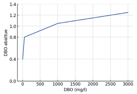
Figure 2 : Abatement de la DBO5 par rapport à la concentration dans le RAC
