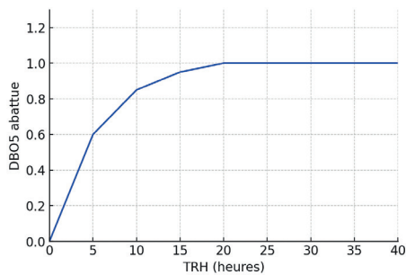
Figure 5 : Abatement de la DBO5 par rapport au TRH dans le RAC
